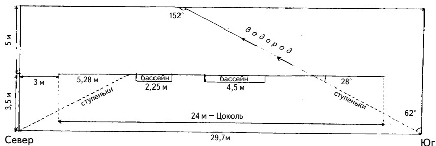
Получение водородной плазмы.
