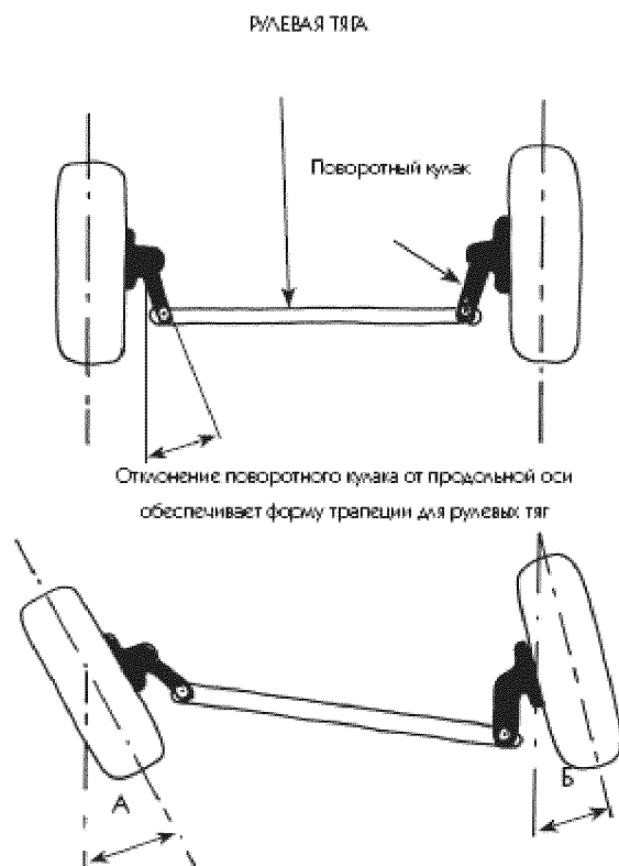
Угол поворота внутреннего колеса больше, чем угол внешнего: A > B Рис.
