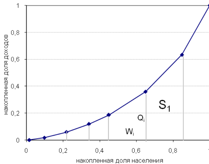
Рис. 2 Графическое представление коэффициента Джини
