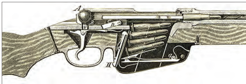
Система Манлихера образца 1886 года (М1886 калибра 11х58 мм R и М1886-90 калибра 8х52 R)
