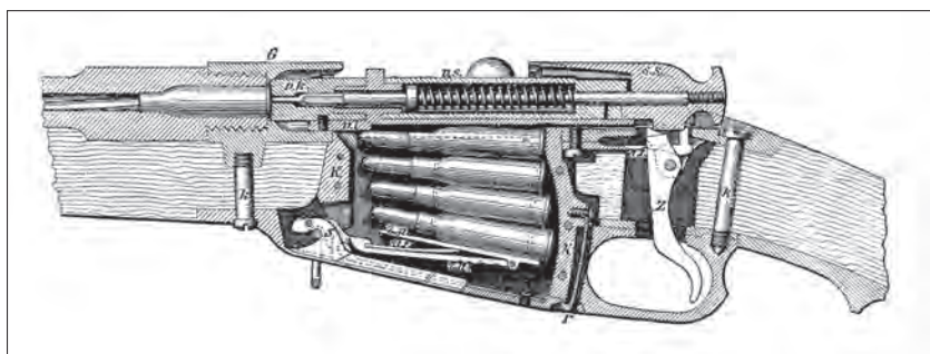
Система 7,62-мм винтовки Мосина обр. 1891 г. (1891/1930 гг.)
