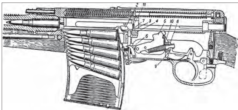
Система самозарядной винтовки Токарева СВТ-38/40 АВТ-40
