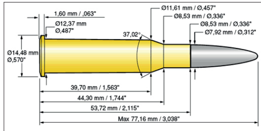
Патрон 7,62x54мм R 305 , 1891, Россия
