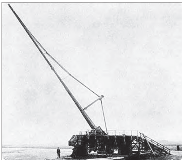
Сверхдальнобойная пушка «Колоссаль»
