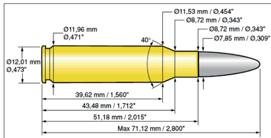
Патрон 7,62x51 мм /.308 Winchester, 1947, США
