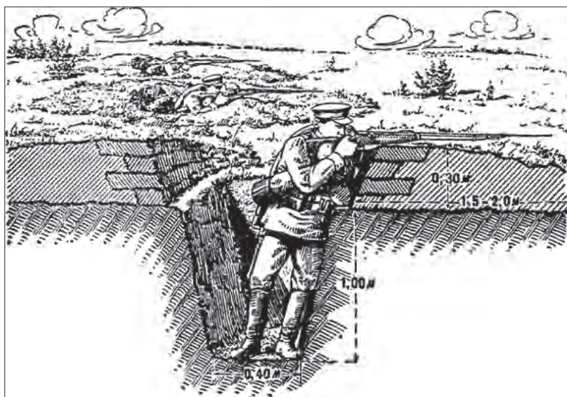
Линия индивидуальных окопов
