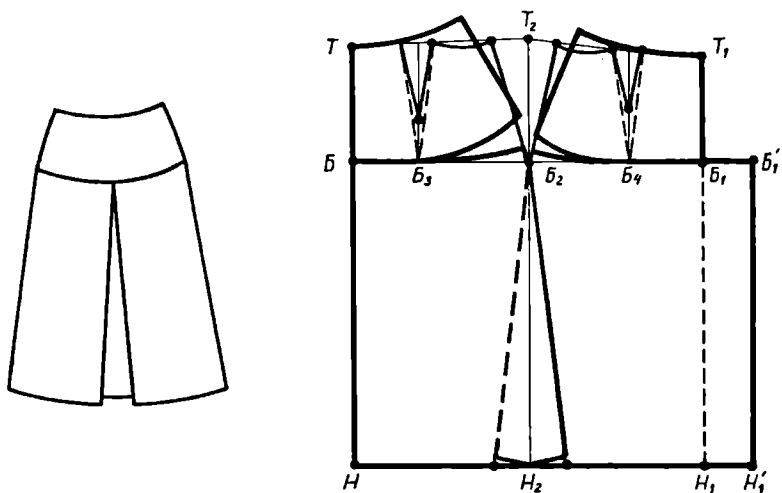
Рис. 21. Техническое моделирование формы юбки.
