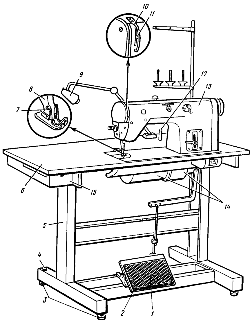
Рис. 45. Швейная машина с промышленным столом.
