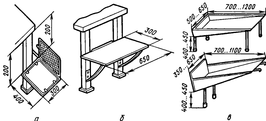
Рис. 39. Откидная подставка (а), выдвижной стеллаж (б) и скаты (в)
