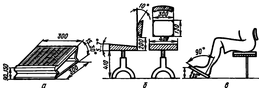
Рис. 2. Приспособления для создания оптимальной рабочей позы «сидя»:
