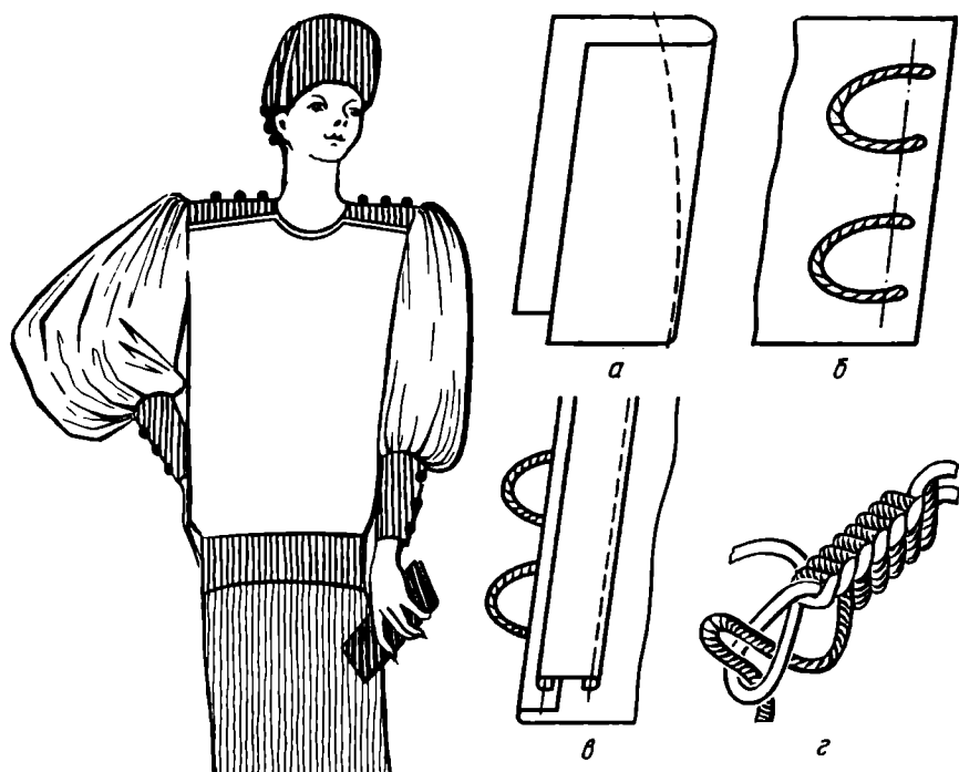
Рис. 72. Обработка петель из вытачного и плетеного шнура.
