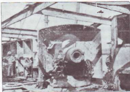
... пробоина в щите 5,5-дм орудия
