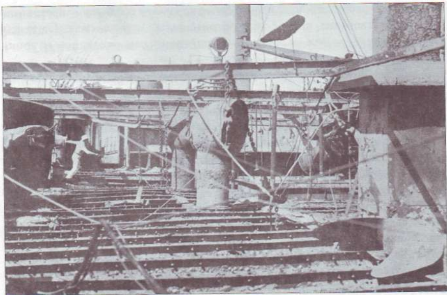
Испанский крейсер «Инфанта Мария Тереза» после боя у Сантьяго: бимсы и остатки сгоревшей палубы правого борта (вверху),
