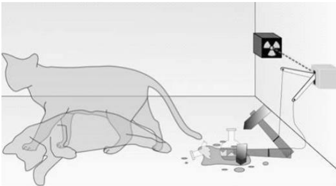
Рис. 2.7. Парадокс кота Шрёдингера.
