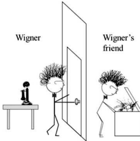
Рис. 2.8. Парадокс друга Вигнера ([13]).
