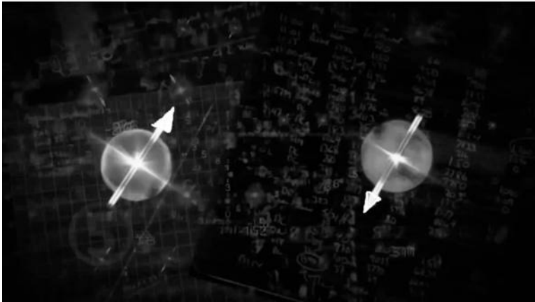
Рис. 2.11. Две частицы с противоположно ориентированными спинами ([7]).
