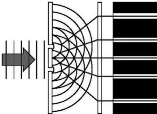
Рис. 2.4. Полосы на детекторе, образующиеся при прохождении волн через две щели ([8]).
