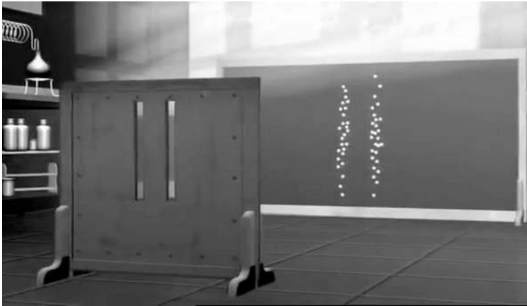
Рис. 2.2. Полосы на детекторе, образующиеся напротив каждой из щелей при пролёте твёрдых тел ([7]).
