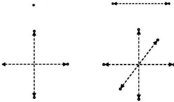
Рис. 4.3. Геометрический подход. Случаи с количеством степеней свободы n=0,1,2,3 . При этом случай n=0 (точка) соответствует нерексорирующему ИС.
