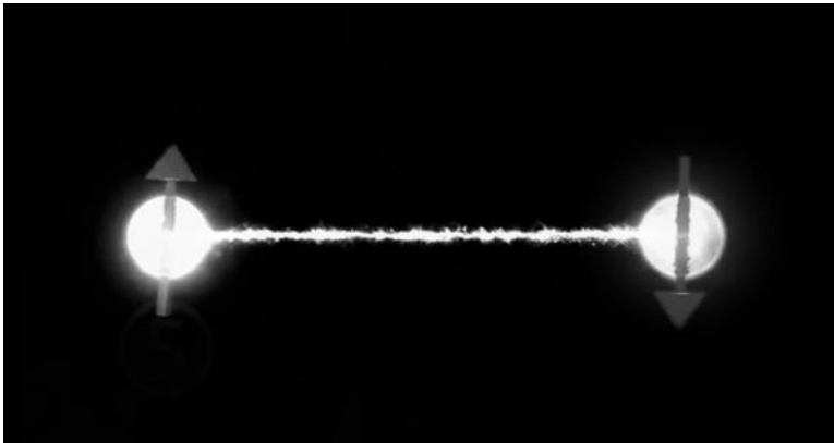
Рис. 2.12. Нелокальная связь ([7]).
