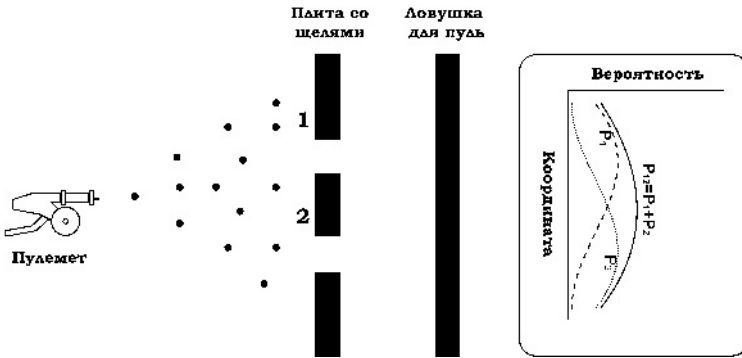
Рис. 2.1. Распределение попаданий на детекторе в случае одиночных частиц или твёрдых тел ([6]).
