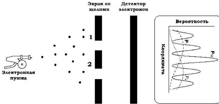
Рис. 2.3. Интерференционная картина на детекторе, полученная после прохождения электронов через две щели ([6]).
