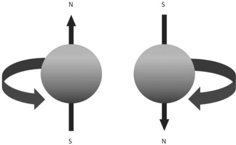
Рис. 2.10. Спин как направление вращения частицы ([15]).
