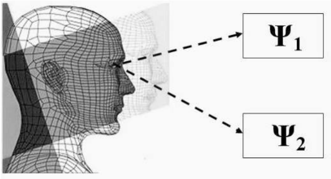
Рис. 2.6. Квантовая суперпозиция, или «наложение» двух состояний.
