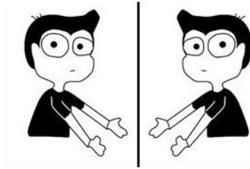
Рис. 4.2. Ауторефлексивная двойственность.
