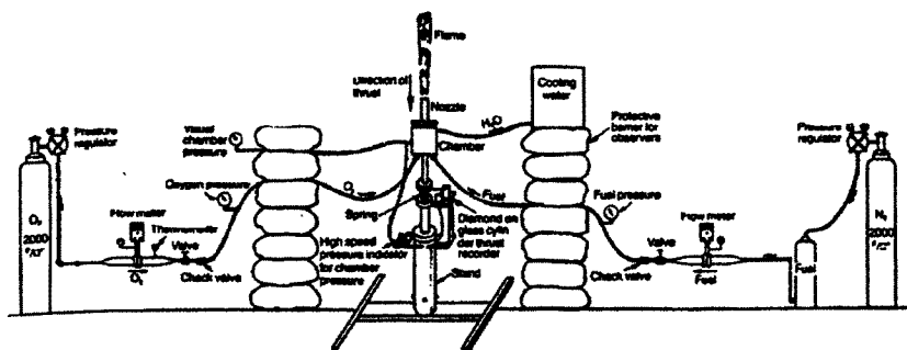
Схематический чертёж испытательной установки для исследования ракеты CALCIT, выполненный Фрэнком Малиной в августе 1936 г.
