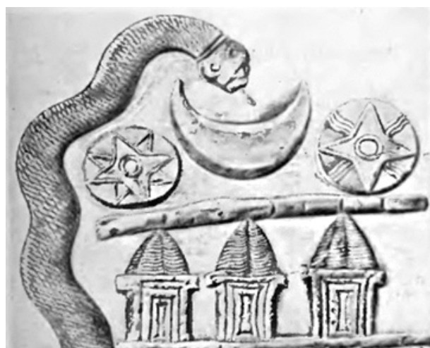
Венера, Земля и Луна.
