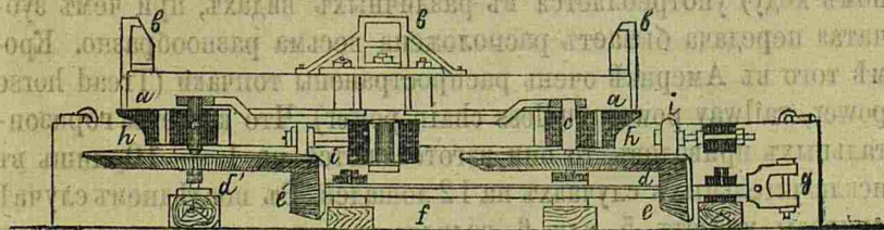
Вертикальный разръзъ.
