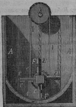
Разрѣзъ прибора для сбиванія масла.
