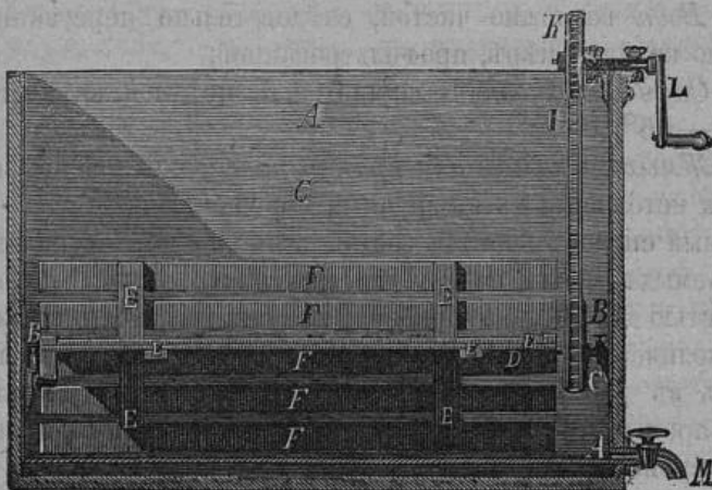
Приборъ для сбиванія масла.
