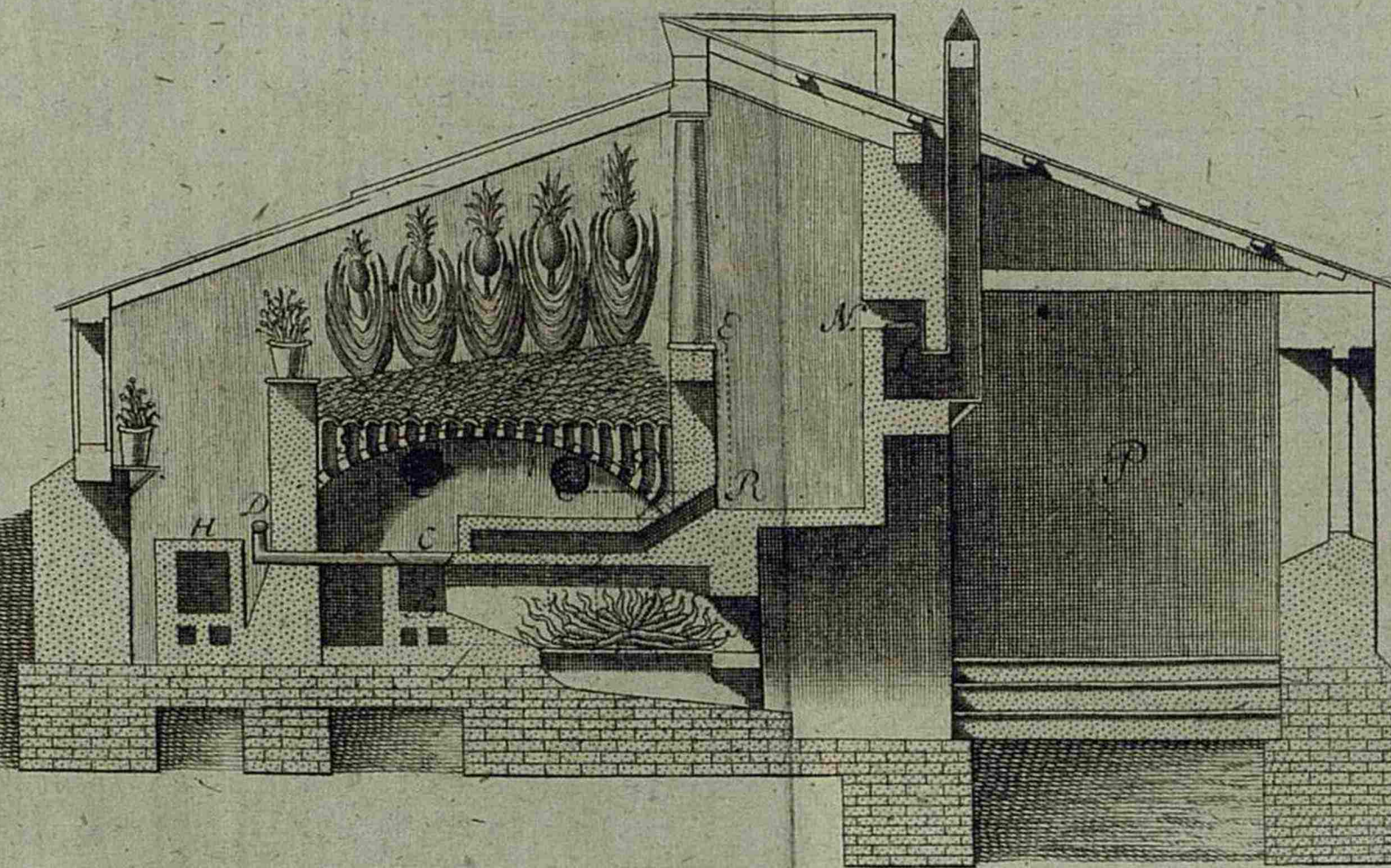
фиг: II. прорѣзъ паровой теплицы.
