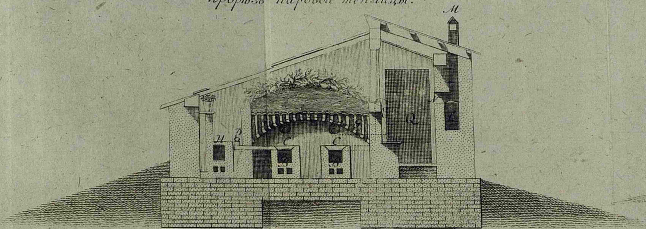
фиг. II. прорѣзъ паровой теплицы.
