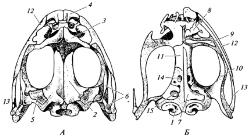
Рис. 70. Череп лягушки:
