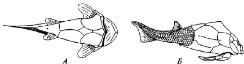
Рис. 62. Панцирные рыбы:
