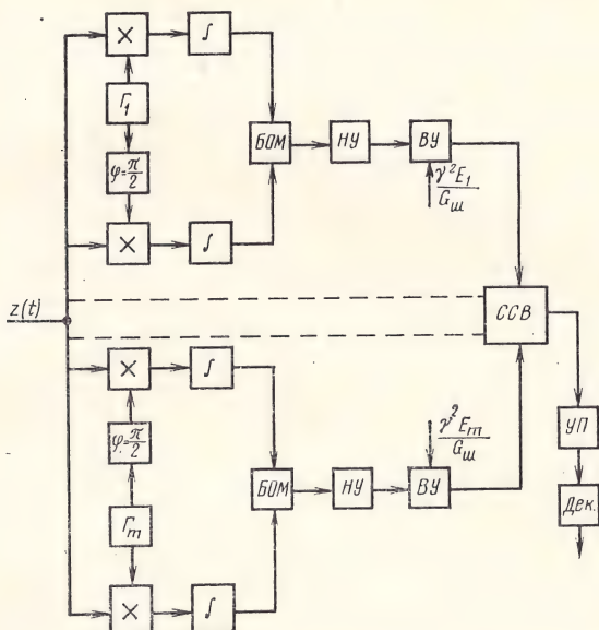
Рис. 5.18. Структурная схема оптимального по критерию максимального правдоподобия приемника при неопределенной фазе сигнала (квадратурная схема)
