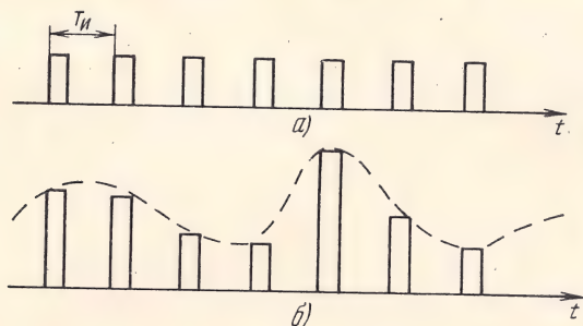
Рис. 6.6. Импульсный переносчик (а) и реализация сигнала АИМ (б)
