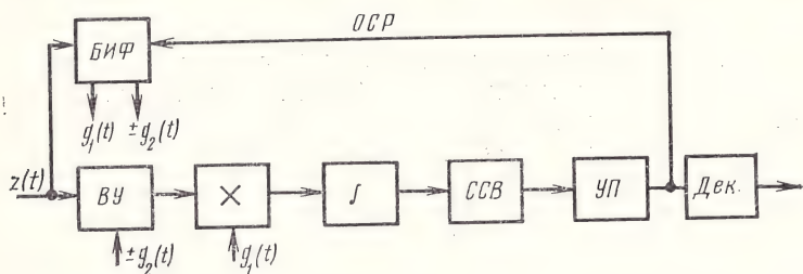
Рис. 5.10. Структурная схема оптимального приемника двоичных сигналов для канала с памятью
