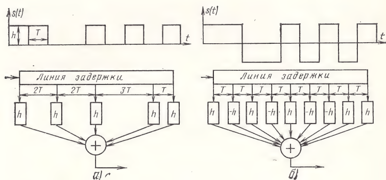
Рис. 5.15. Реализация согласованных фильтров на основе линии задержки:
