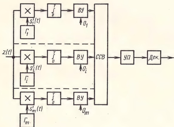
Рис. 5.5. Структурная схема корреляционного приемника при точно известном ансамбле сигналов
