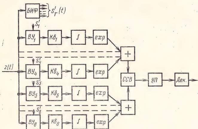
Рис. 5.8. Структурная схема оптимального приемника для канала с памятью
