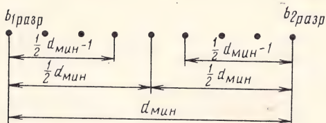
Рис. 4.3. К оценке обнаруживающей и исправляющей способности корректирующего кода
