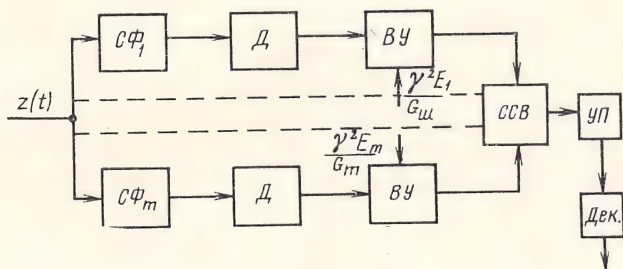
Рис. 5.19. Реализация оптимального по критерию максимального правдоподобия приемника при неопределенной фазе сигнала на базе согласованных фильтров
