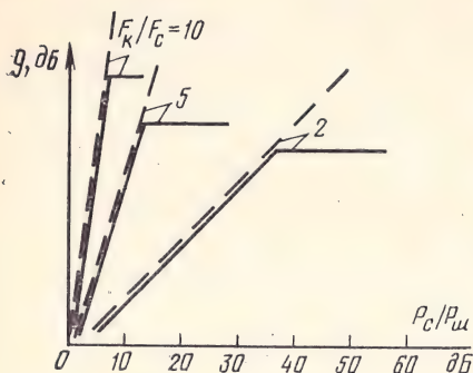
Рис. 6.8. Зависимость выигрыша системы модуляции от отношения сигнал/шум в канале: — — — — — для идеальной системы; ————— для реальной системы
