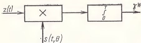
Рис. 6.2. Структурная схема оптимального измерителя коэффициента передачи канала при точно известном сигнале
