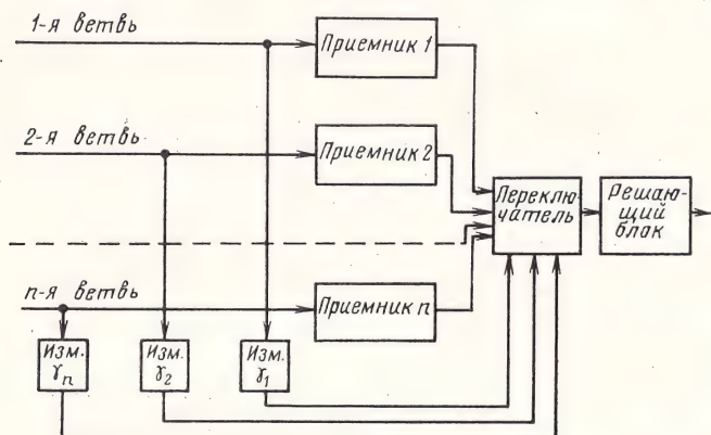
Рис. 5.20. Схема разнесенного приема с автовыбором ветви с наиболее сильным сигналом
