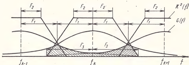
Рис. 7.1. К определению переходной помехи и разноса между канальными частотами многоканальной системы при трапециевидных характеристиках разделительных фильтров
