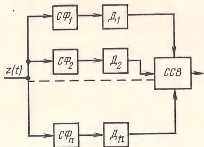
Рис. 6.5. Структурная схема оптимального измерителя частоты при неопределенной фазе сигнала
