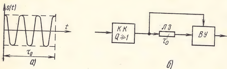
Рис. 6.16. Прямоугольный радиоимпульс (а) и согласованный с ним фильтр (б)
