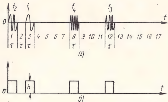
Рис. 7.8. Канальный сигнал асинхронно-адресной системы связи (а) и сигналы на выходе амплитудных детекторов (б)
