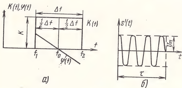
Рис. 6.15. Частотные характеристики идеального полосового фильтра (а) для прямоугольного радиопульса (б)
