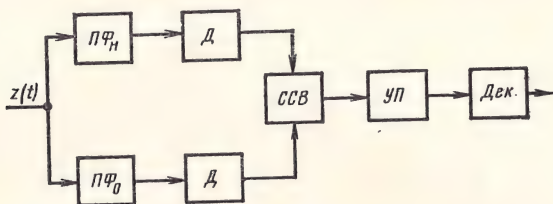
Рис. 5.17. Структурная схема неоптимального приема сигналов ЧМ методом сравнения огибающих в разделительных фильтрах
