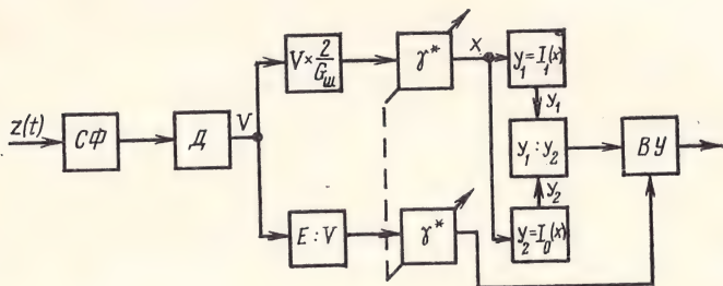
Рис. 6.3. Структурная схема оптимального измерителя коэффициента передачи канала при неопределенной фазе сигнала
