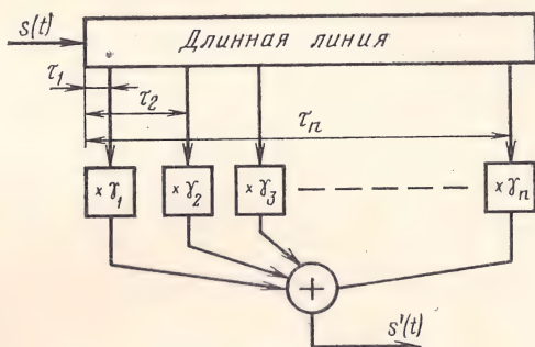
Рис. 2.3. Модель многолучевого канала
