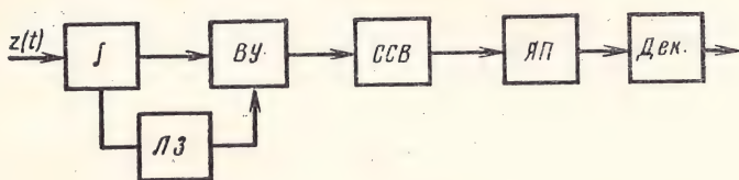
Рис. 5.12. Структурная схема оптимального приемника с согласованным фильтром для одиночного прямоугольного импульса
