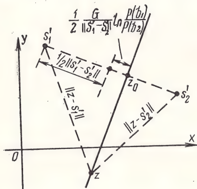
Рис. 5.7. К оптимальному разбиению пространства трех сигналов по критерию идеального наблюдателя
