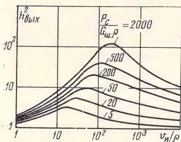
Рис. 6.11. Зависимость отношения сигнал/шум на выходе системы ДМ от величины v_{\text{и}}/\rho
