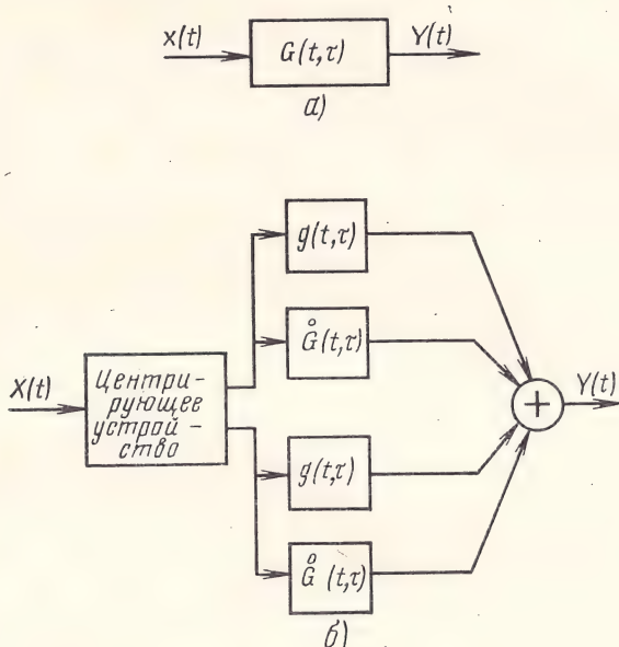
Рис. 2.5. Прохождение случайных воздействий через линейную систему со случайно меняющимися параметрами:
