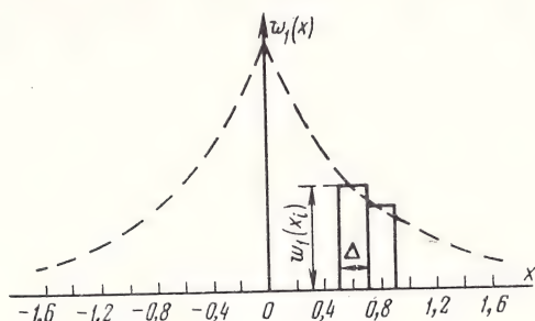
Рис. 3.2. К определению вероятностей появления уровней квантованного сигнала
