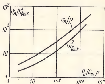
Рис. 6.12. Зависимость максимальной величины h_{\text{вых}}^2 и оптимальной величины v_{\text{и}}/\rho от P_c/G_{\text{ш}}\rho для системы ДМ
