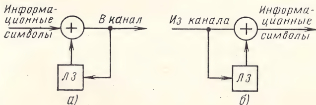
Рис. 4.6. Структурные схемы кодера (а) и декодера (б) для относительного кода
