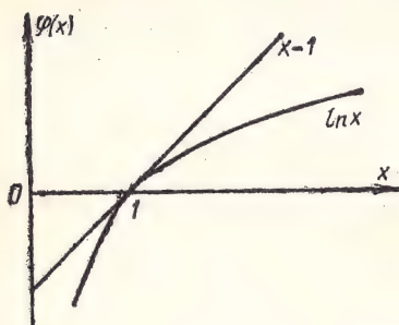
Рис. 3.1. К пояснению неравенства \ln x \leq x-1
