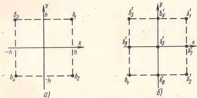
Рис. 1.6. Пространство сигналов на передаче (а) и приеме (б) при наличии стираний
