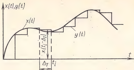
Рис. 1.3. К пояснению восстановления непрерывного процесса X(t) путем формирования ступенчатой функции
