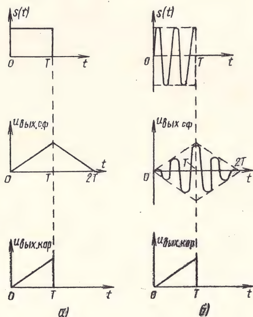
Рис. 5.16. Диаграммы напряжений на выходе коррелятора и согласованного фильтра при подаче на вход прямоугольных видеопульса (а) и радиопульса (б)
