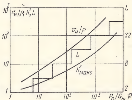
Рис. 6.10. Зависимость максимальной величины h_{\text{вых}}^2 и оптимальных значений v_n/\rho и L от P_c/G_{\text{ш}}\rho для системы КИМ
