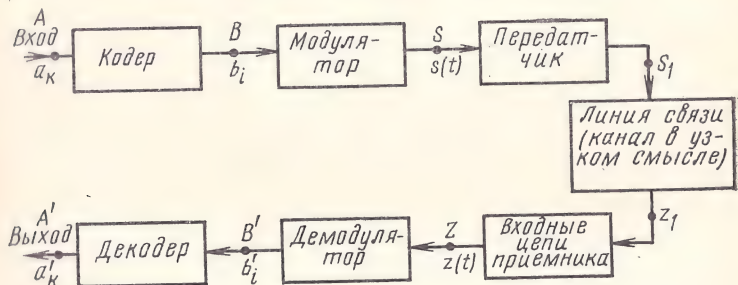
Рис. 2.1. Структурная схема канала связи при передаче дискретных сообщений
