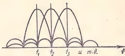
Рис. 7.7. Амплитудный спектр группового сигнала многоканальной системы связи с ортогональными сигналами МС-5
