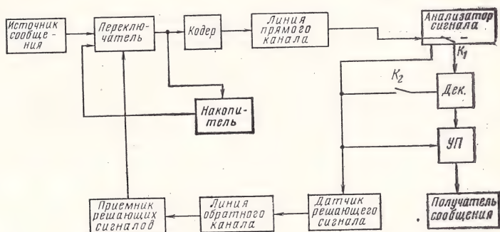
Рис. 5.21. Структурная схема дискретной системы с управляющей обратной связью
