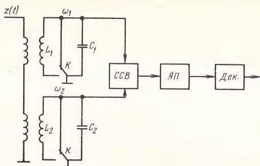
Рис. 5.13. Реализация оптимального по критерию максимального правдоподобия приемника сигналов ЧМ на базе согласованных фильтров
