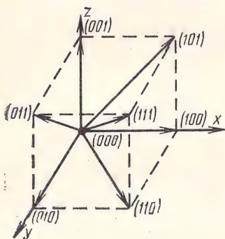
Рис. 1.4. Представление трехразрядных двоичных сигналов в трехмерном пространстве
