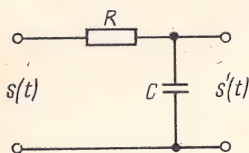
Рис. 2.2. Модель линейного канала с постоянными параметрами
