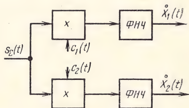
Рис. 7.4. Структурная схема приемного устройства двухканальной системы связи с фазовым уплотнением
