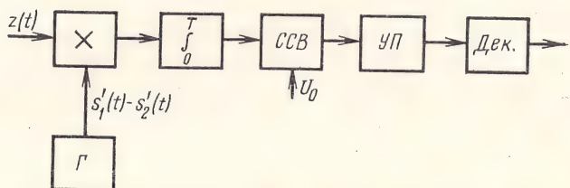
Рис. 5.6. Структурная схема корреляционного приемника для двоичных сигналов
