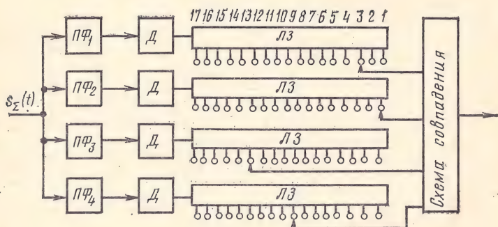
Рис. 7.6. Структурная схема приемного устройства асинхронно-адресной системы связи
