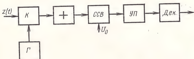
Рис. 5.3. Структурная схема оптимального приемника по трем отсчетам при точно известном сигнале
