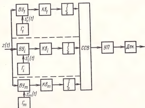
Рис. 5.4. Реализация оптимального приемного устройства по критерию максимального правдоподобия при точно известном ансамбле сигналов
