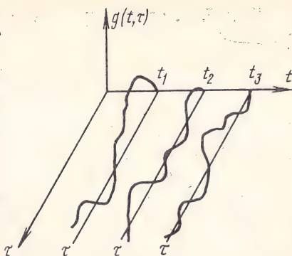
Рис. 2.4. Реализации импульсных переходных характеристик линейного канала со случайно меняющимися параметрами
