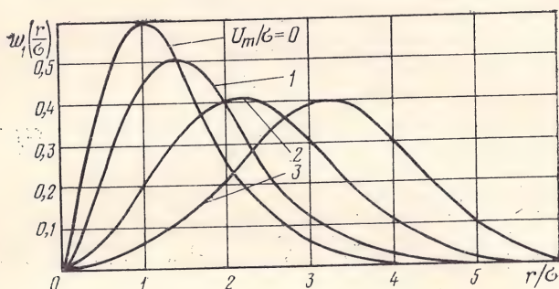
Рис. 1.2. Обобщенно-рэлеевское распределение огибающей узкополосного нормального случайного процесса
