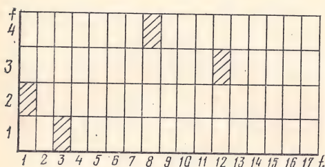
Рис. 7.5. Частотно-временная матрица
