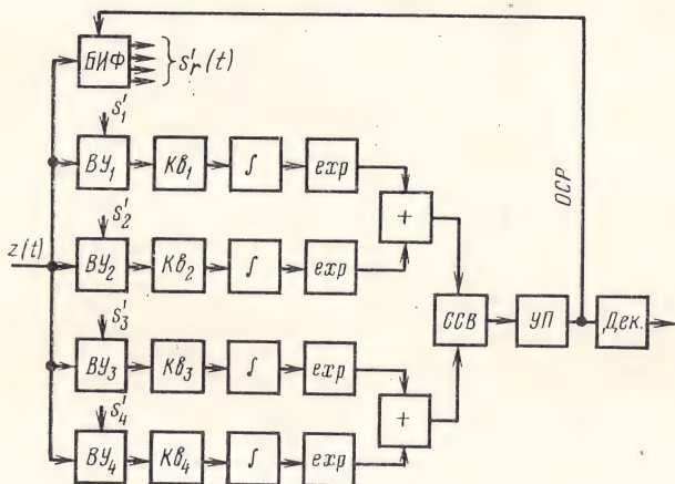
Рис. 5.9. Структурная схема приемника с обратной связью по решению
