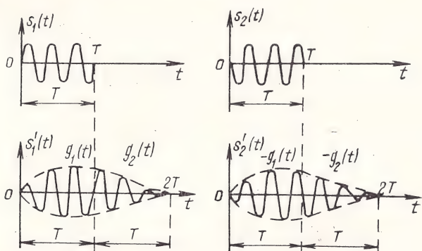
Рис. 5.1. Сигналы ФМ на входе и выходе канала с памятью
