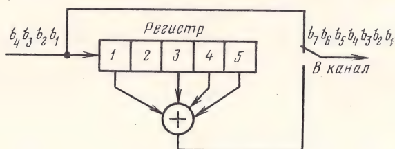
Рис. 4.2. Схема формирования двоичного кода
