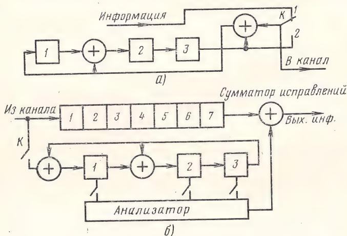
Рис. 4.4. Структурные схемы кодера (а) и декодера (б) циклического кода (7,4)
