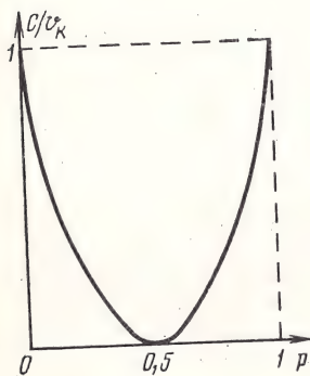
Рис. 3.4. Зависимость нормированной пропускной способности двоичного симметричного канала без памяти от вероятности ошибочного приема символа
