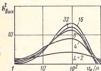
Рис. 6.9. Зависимость отношения сигнал/шум на выходе системы КИМ от величины v_n/\rho при различном числе уровней квантования
