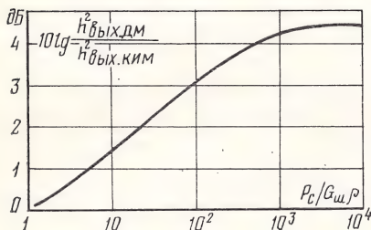
Рис. 6.13. Зависимость энергетического выигрыша перехода от системы КИМ к системе ДМ от величины P_c/G_{\text{шр}}
