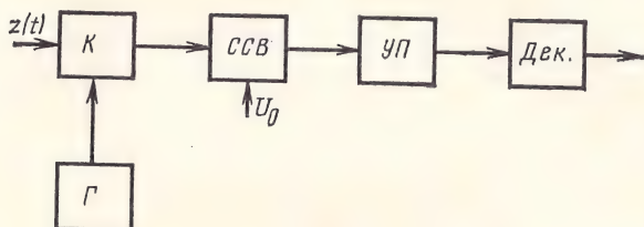
Рис. 5.2. Структурная схема оптимального приемника по одному отсчету при точно известном сигнале
