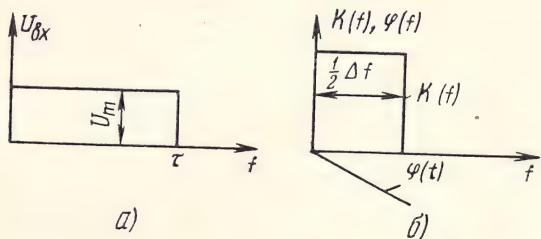
Рис. 6.17. Огибающая прямоугольного радиоимпульса (а) и частотная характеристика идеального ФНЧ (б)
