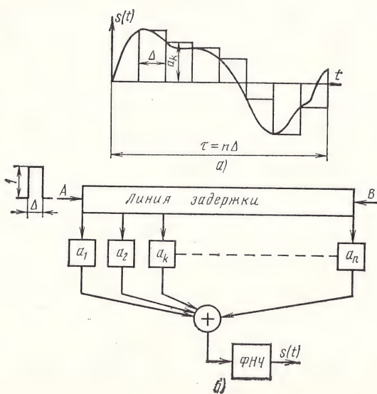
Рис. 5.14. Реализация фильтра, согласованного с произвольным непрерывным сигналом, на основе линии задержки с отводами и блоками взвешивания:
