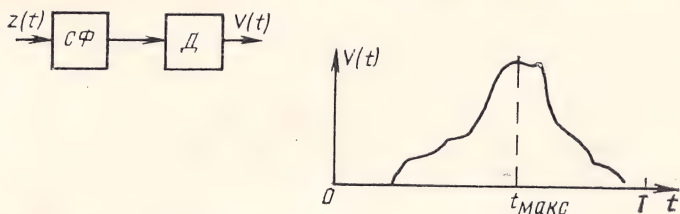
Рис. 6.4. Оптимальный измеритель времени прихода сигнала с неопределенной фазой
