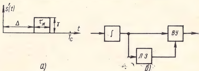
Рис. 6.14. Прямоугольный импульс (а) и согласованный с ним фильтр (б)
