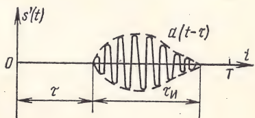
Рис. 6.1. К определению оптимальной оценки времени прихода сигнала
