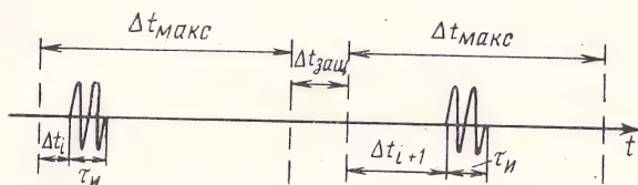
Рис. 7.2. Реализация сигнала многоканальной системы связи с фазо-импульсной модуляцией
