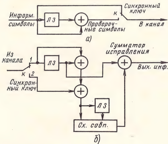
Рис. 4.5. Структурные схемы кодера (а) и декодера (б) для рекуррентного кода (1/2)
