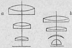
Рис. 1. Схемы объектива сложного микроскопа (а—прежней, б—новой конструкции).
