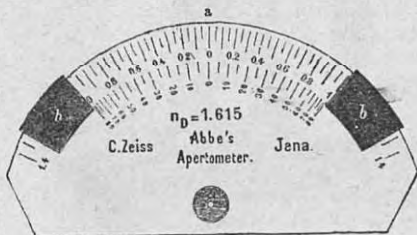
Рис. 7. Аперетометръ Аббе.
