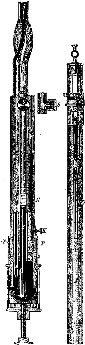
Рис. 1. Барометръ Вильда-Фюсса.
