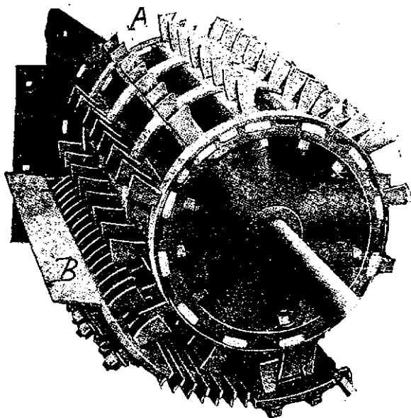
Рис. 3. Открытый штифтовый барабан; А — барабан, В — подбарабанье.
