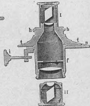
Къ рис. 10. Поляризационное приспособленіе: I—анализаторъ; t и n—кулачки съ дѣленіями; i—винтъ, неподвижно закрѣпляющій f и n въ трубѣ микроскопа; II—поляризаторъ.
