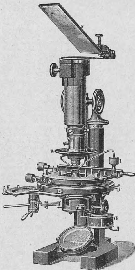
Рис. 10. Микроскоп Цейсса: g —приспособление для согревания, l —воздушное охлаждение, p , a —поляризатор и анализатор, s —зеркало для проектирования.
