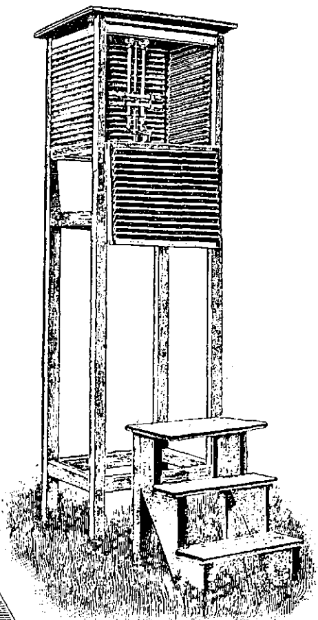
Рис. 12. Будка анемометрическаго образца.
