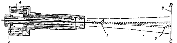
1—расплавленный конец проволоки; 2—частицы расплавленного металла; 3—суживаемый предмет; 4—сжатый воздух; 5—кислородо-водородная смесь.
