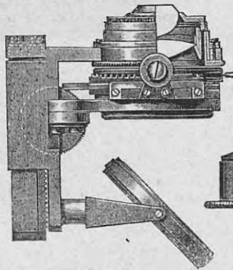
Рис. 6. Освѣтительный приборъ Аббе.
