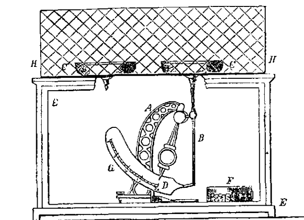
Рис. 9. Испаритель Виаля.
