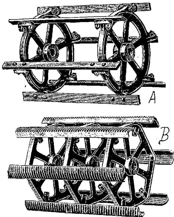
Рис. 1. Бильные барабаны: А — съ гладкими билами, В — съ рифленными билами.
