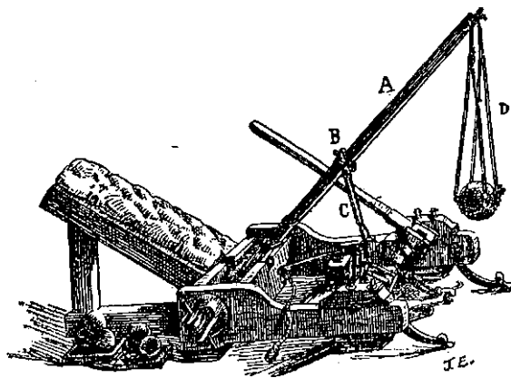
Рис. 1. Онгаръ или механическая праща (по описанію Аммиана Марцеллина).
