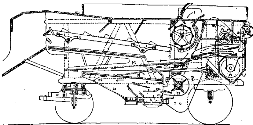
Рис. 4. Разрез сложной молотилки английского оборудования.
