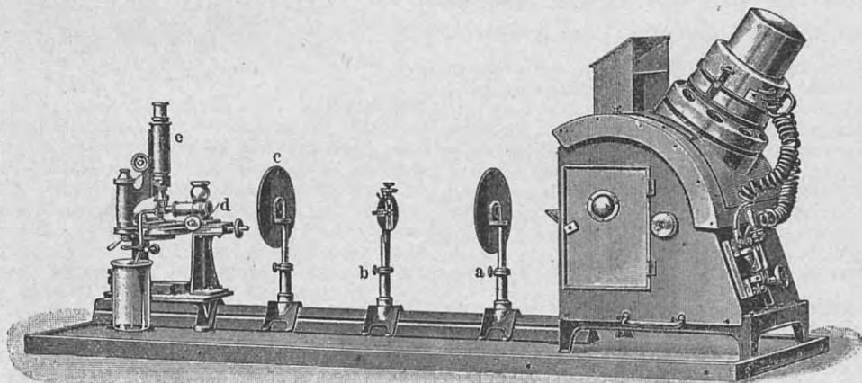
Рис. 11. Ультрамикроскоп (объяснение см. в тексте).
