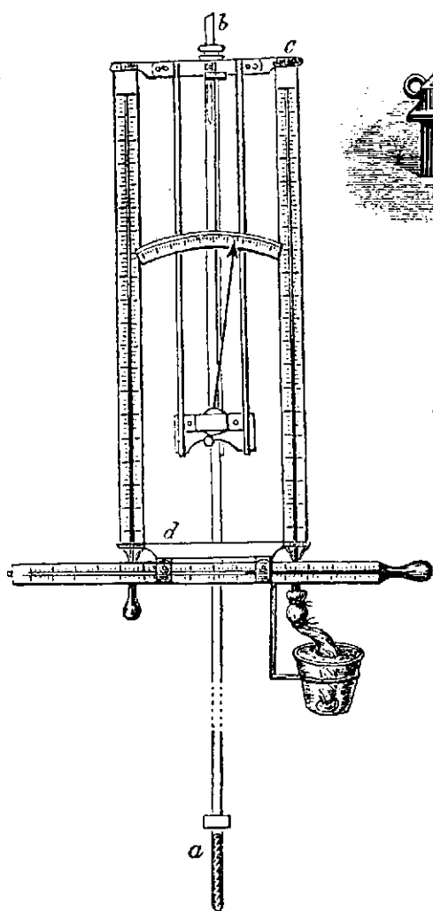
Рис. 3. Установка термометровъ для опредѣленія влажности.
