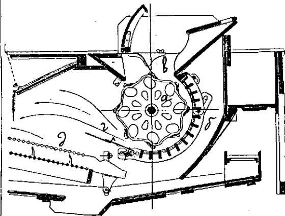
Рис. 2. Бильный барабанъ съ подбарабаньемъ. а — барабанъ; б — дека; в — входъ обмолачиваемаго хлѣба; г — выходъ соломы; д — соломотрясъ.
