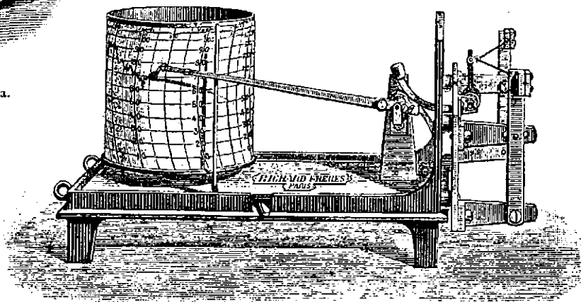
Рис. 5. Гигрографъ Риттера.
