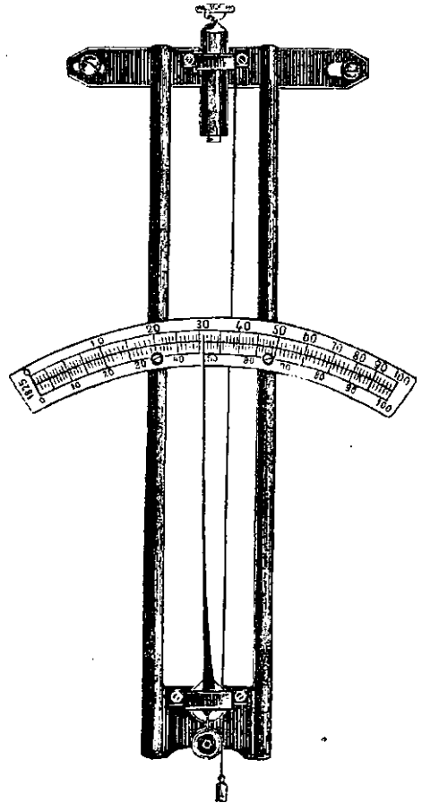
Рис. 2. Барометръ Соссюра.
