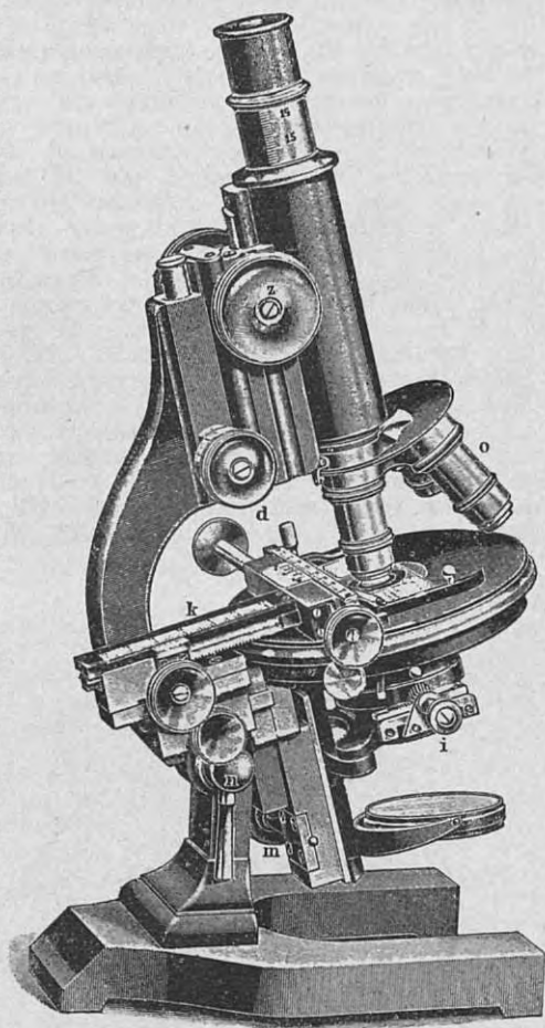
Рис. 9. Большой микроскоп Лейтца: d —винт и z зубчатка для установления микроскопа, i —осветительный прибор, k —столик, m —рычаг, n —шарнир, o —объективный револьвер.
