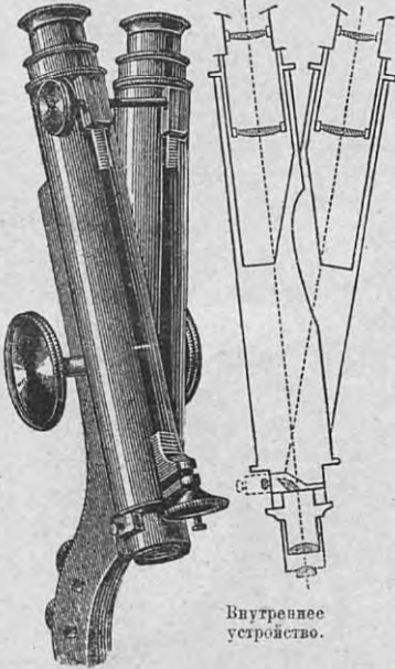
Рис. 4. Бинокулярный микроскопъ Вейссы.
