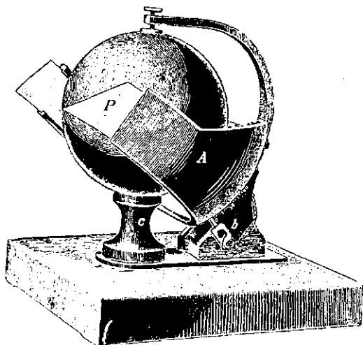
Рис. 8. Гелиографъ Кемпбелля и Стоуна.
