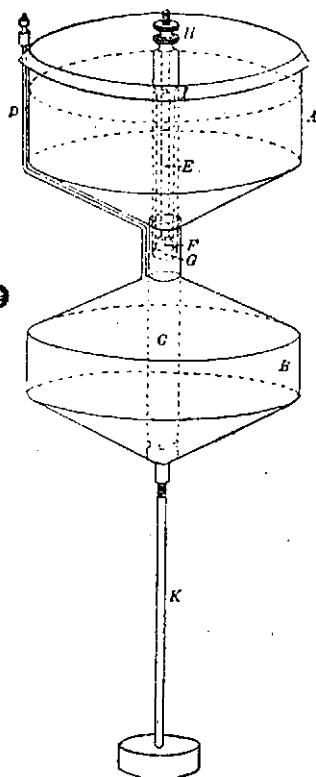
Рис. 6. Испаритель Дерягина-Любославскаго.
