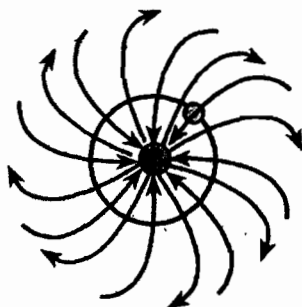
Рис. 6. Схема сепарации (коловращения) в Солнечной системе
