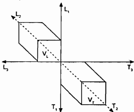
Рис. 9. Система физических величин Р. О. ди Бартини в 6-мерной системе координат
