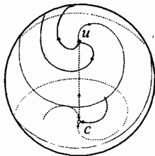
Рис. 10. Строение элементарного осциллятора: u — исток времени — пространства, c — сток
