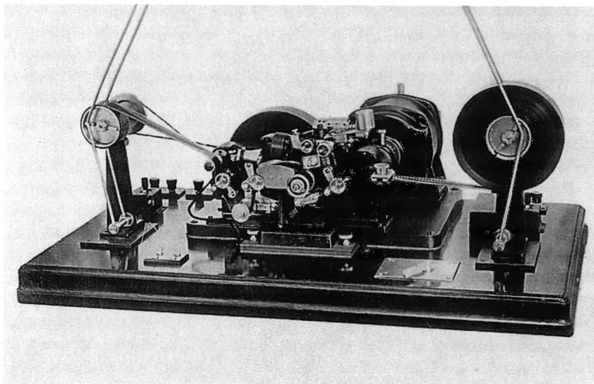
Стационарный шоринофон
