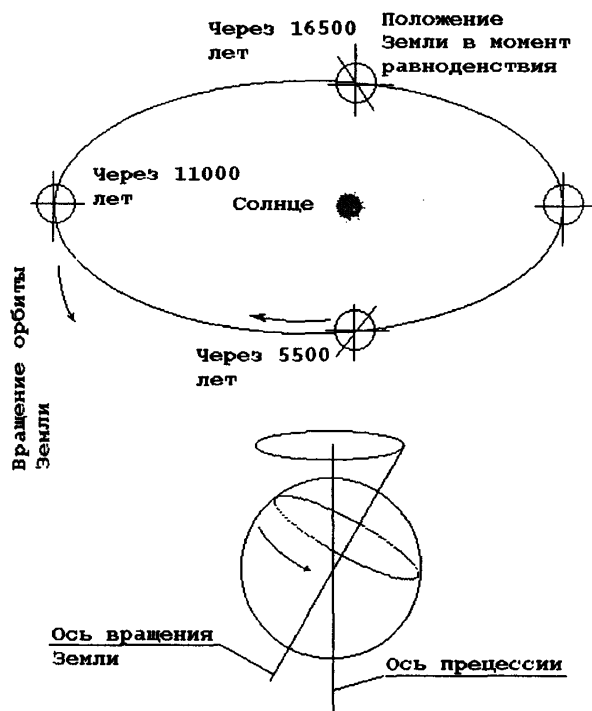
Рис. 20. Предварение равноденствий
